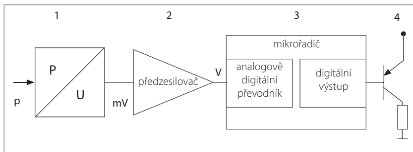
Blokové schéma zapojení
